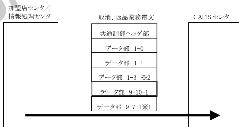
図 2.2-2 取消、返品業務電文構成
