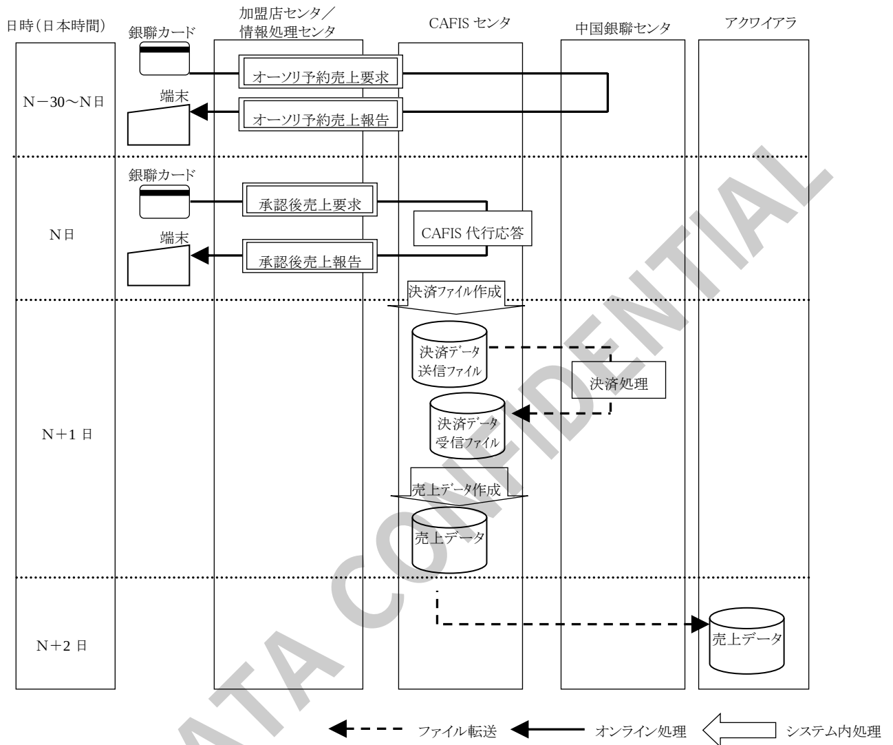
図 2.1-2 オーソリ予約／承認後売上業務処理フロー図
