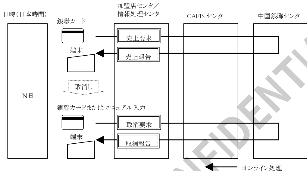
図 2.1-3 取消業務処理フロー図
